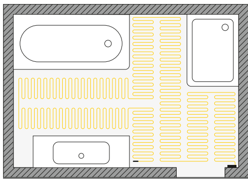
■ TOEPASSING VAN BLANKE ELTOP+ OP HET HELE OPPERVLAK
