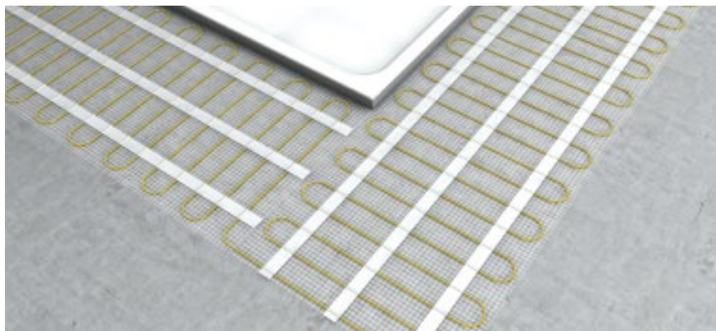
TOEPASSING VAN BLANKE ELOTOP+ IN EEN HOEK VAN 90°
