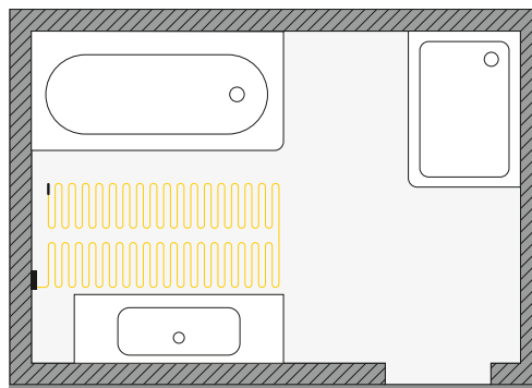
■ TOEPASSING VAN BLANKE ELTOP+ OP EEN DEEL VAN HET OPPERVLAK
